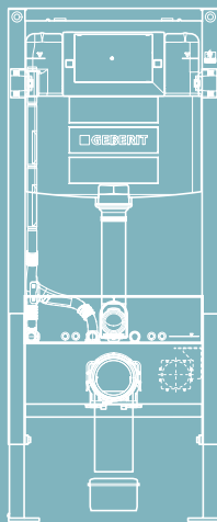
↑ Geberit Omega Unterputz-Spülkasten
